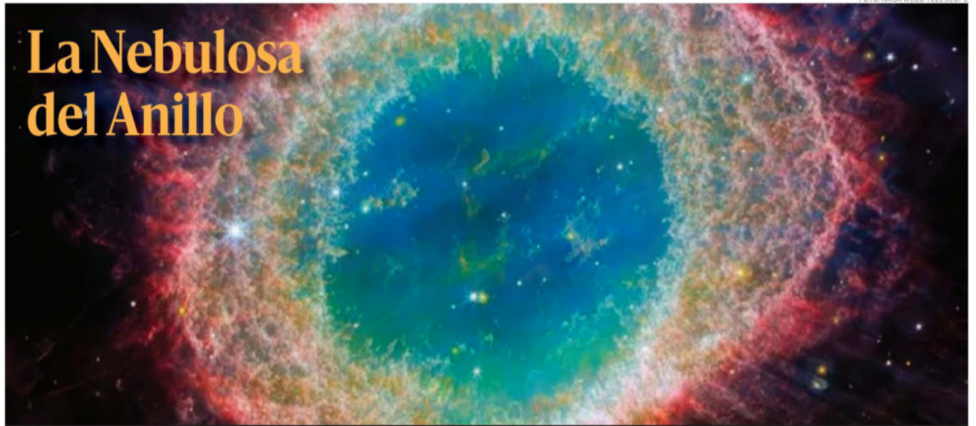
Foto sin precedentes de esta nebulosa, formada de los restos de una estrella en descomposición que se desprende de sus capas externas al quedarse sin combustible, captada por el telescopio espacial James Webb. PAG 23
